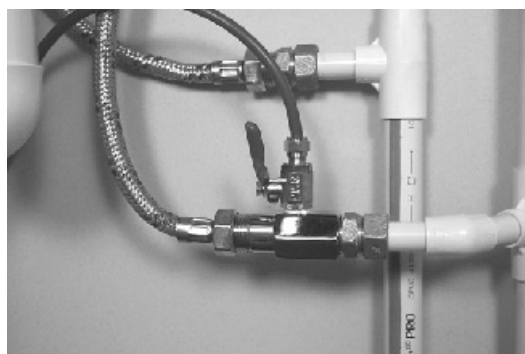
Zdj. 1. Sposób podłączenia zestawu filtrów do instalacji wodociągowej.
